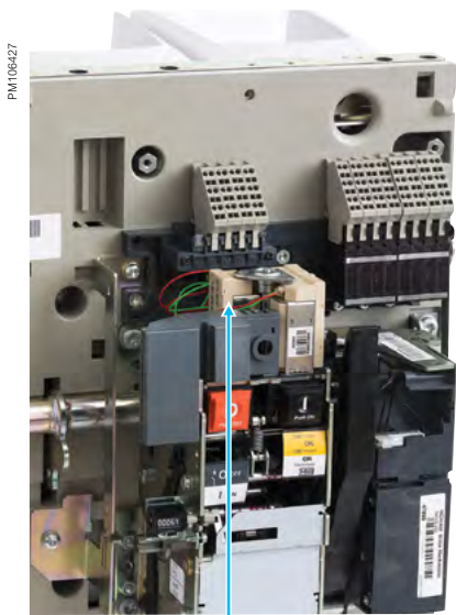
Катушка отключения MX2 или катушка минимального напряжения MN
